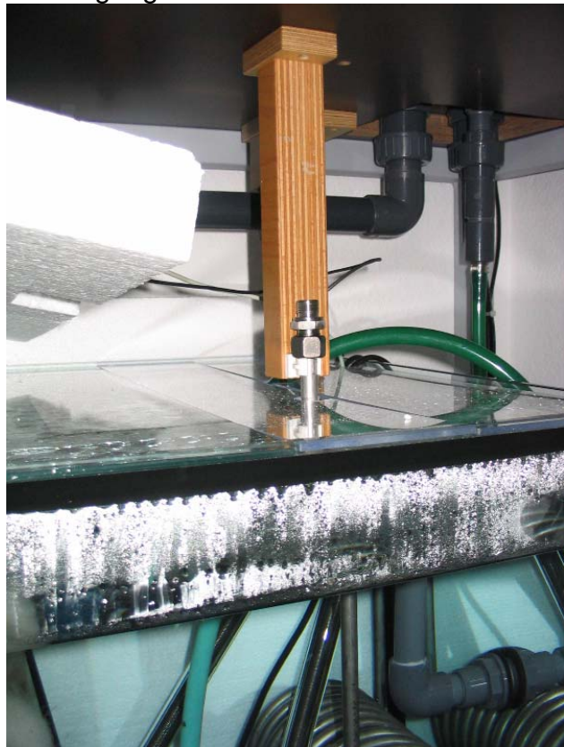
Befestigung Heizwendel
